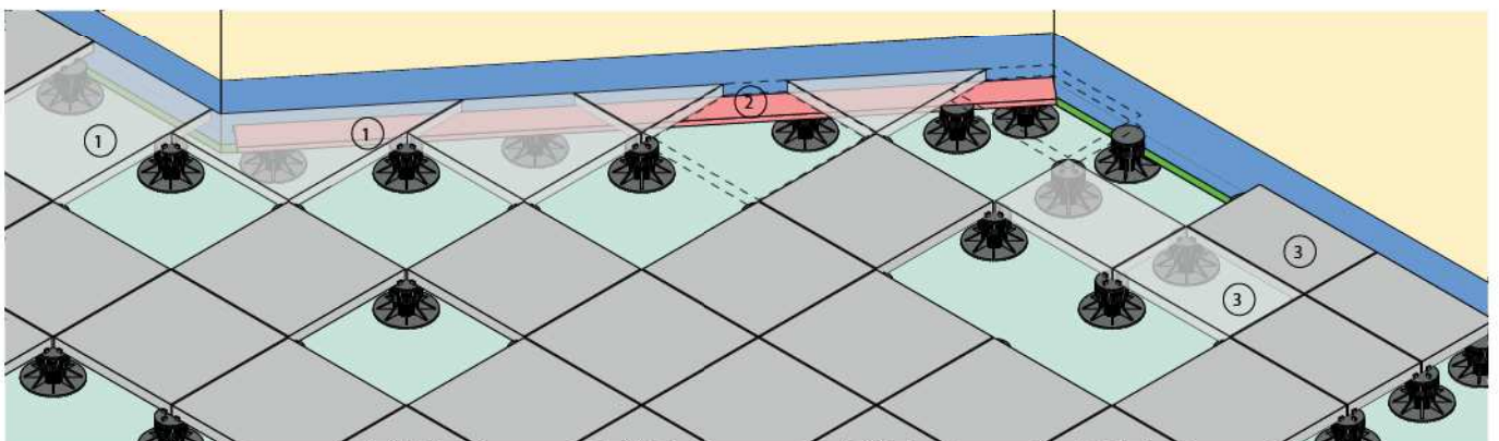
Abb. 8: Anordnung von Stelzlagern unter Anschnittplatten; (1) Anschnittplatten Variante mit grösserem Plattenformat, (2) Metallprofil, (3) Anschluss mit Normalplatten auf 2 oder 3 Plattenreihen verteilt
