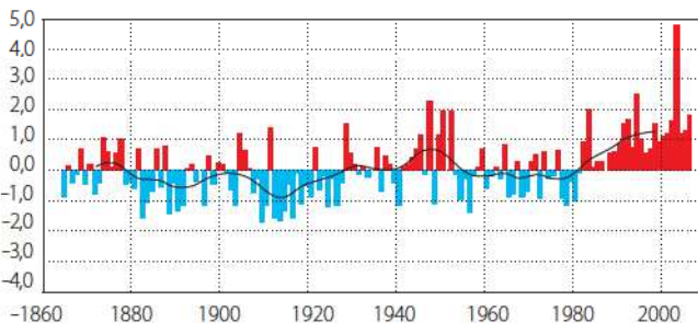
Abb. 1: Mittlere Abweichung der Sommertemperaturen in der Schweiz 1864–2007 von der WMO-Norm 1961–1990; Rot: wärmere Jahre als der Ø von 1961–1990. Blau: kühlere als Ø 1961–1990. (Quelle: MeteoSchweiz)
