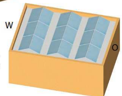
Optimale Flächenausnutzung mit Ost-West ausgerichteten PV-Modulen
